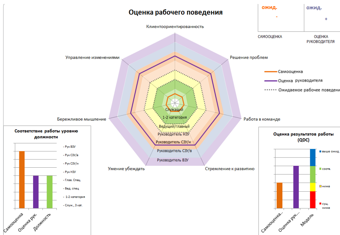
Рисунок 3 — Радар-диаграмма AssessmentProtocol
